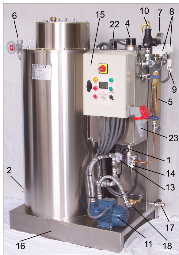
Dampfkessel 150-300
